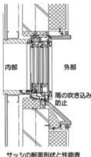
サッシの断面形状と性能表
